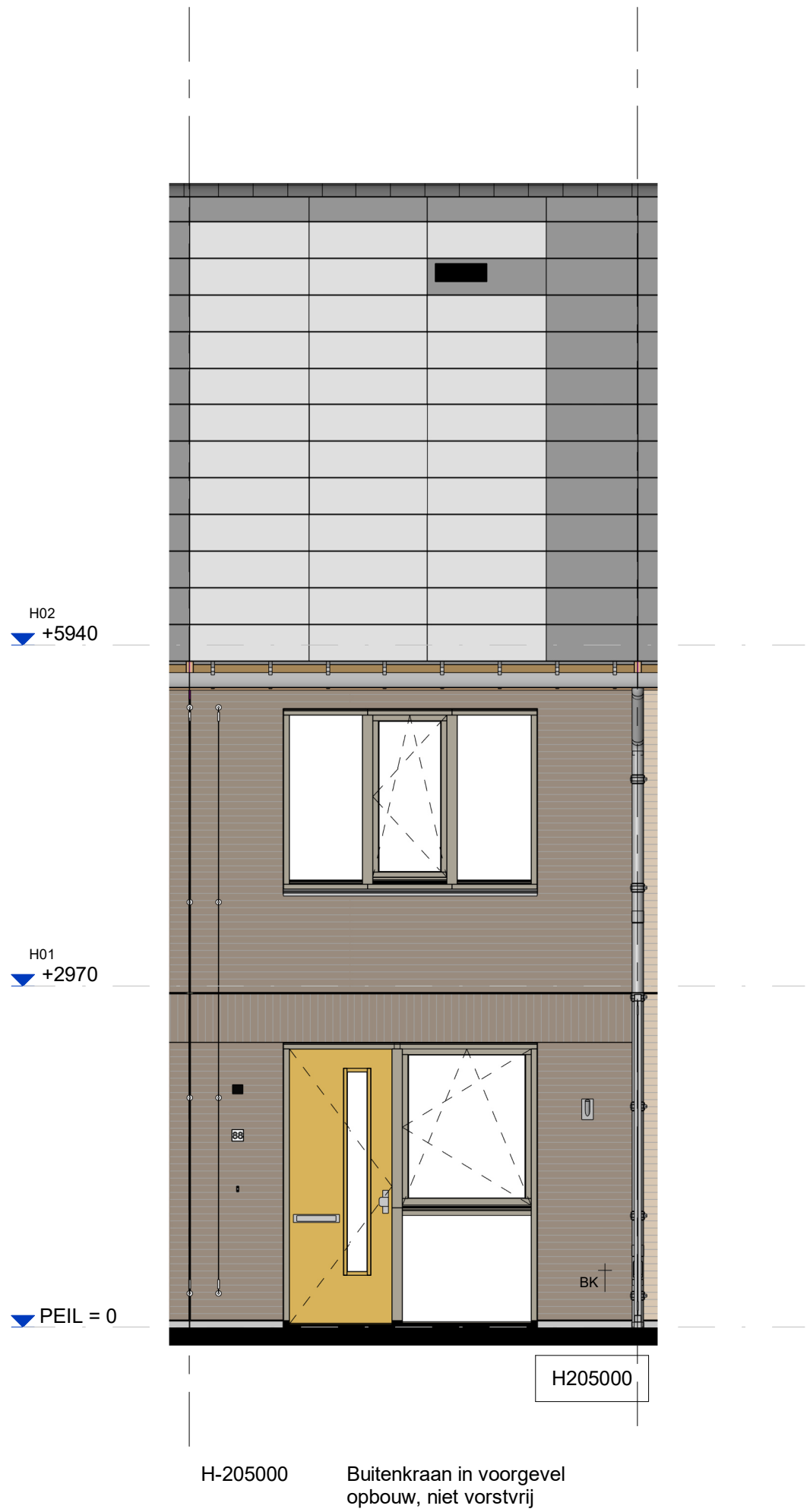
Voorgevel
