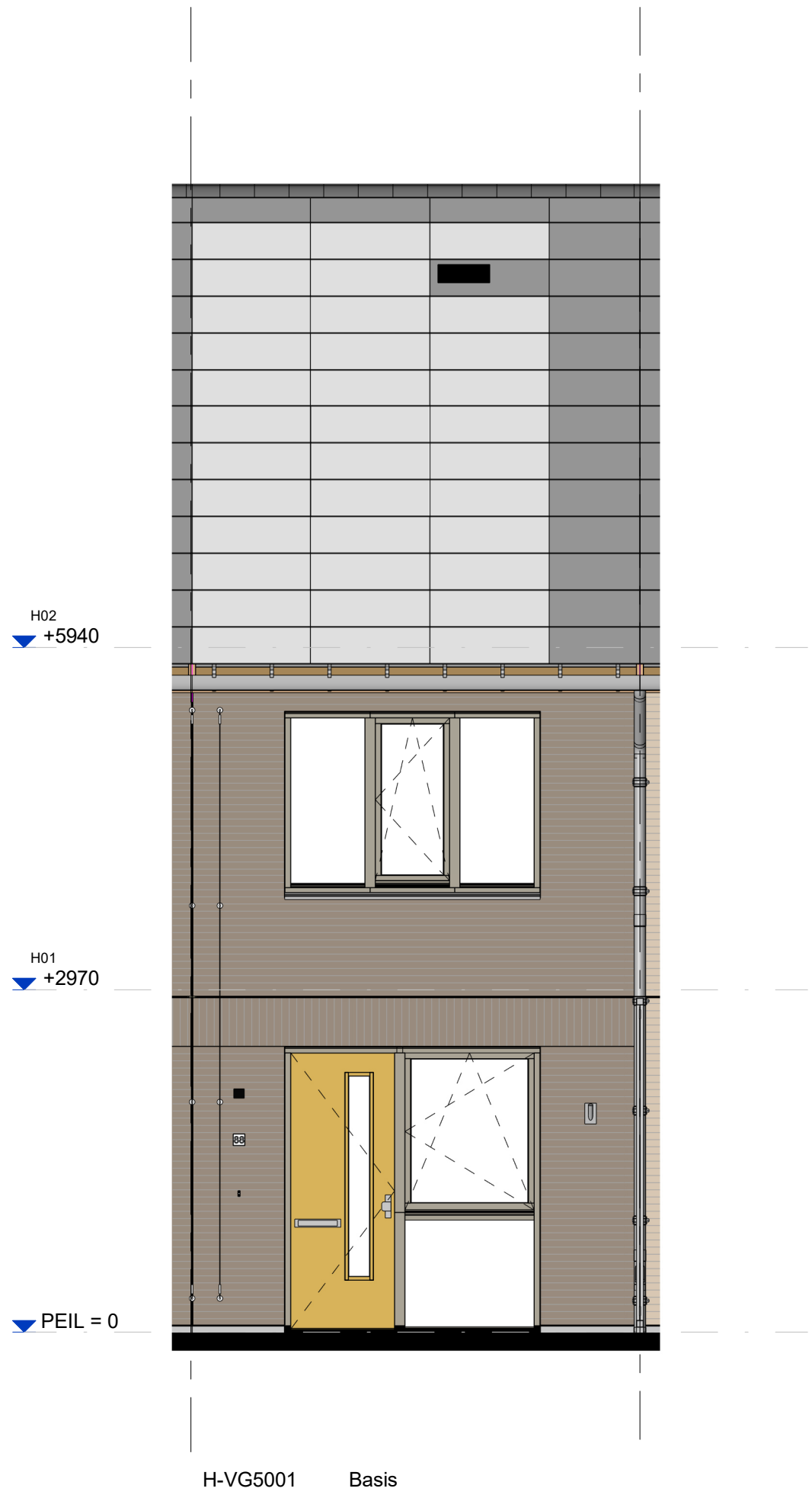
Voorgevel
