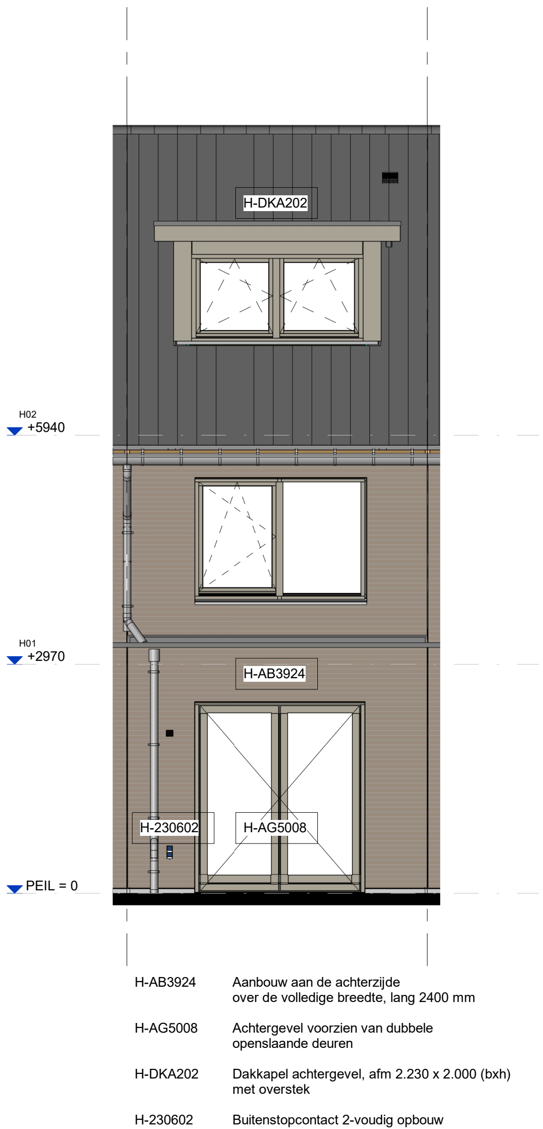
Achtergevel
