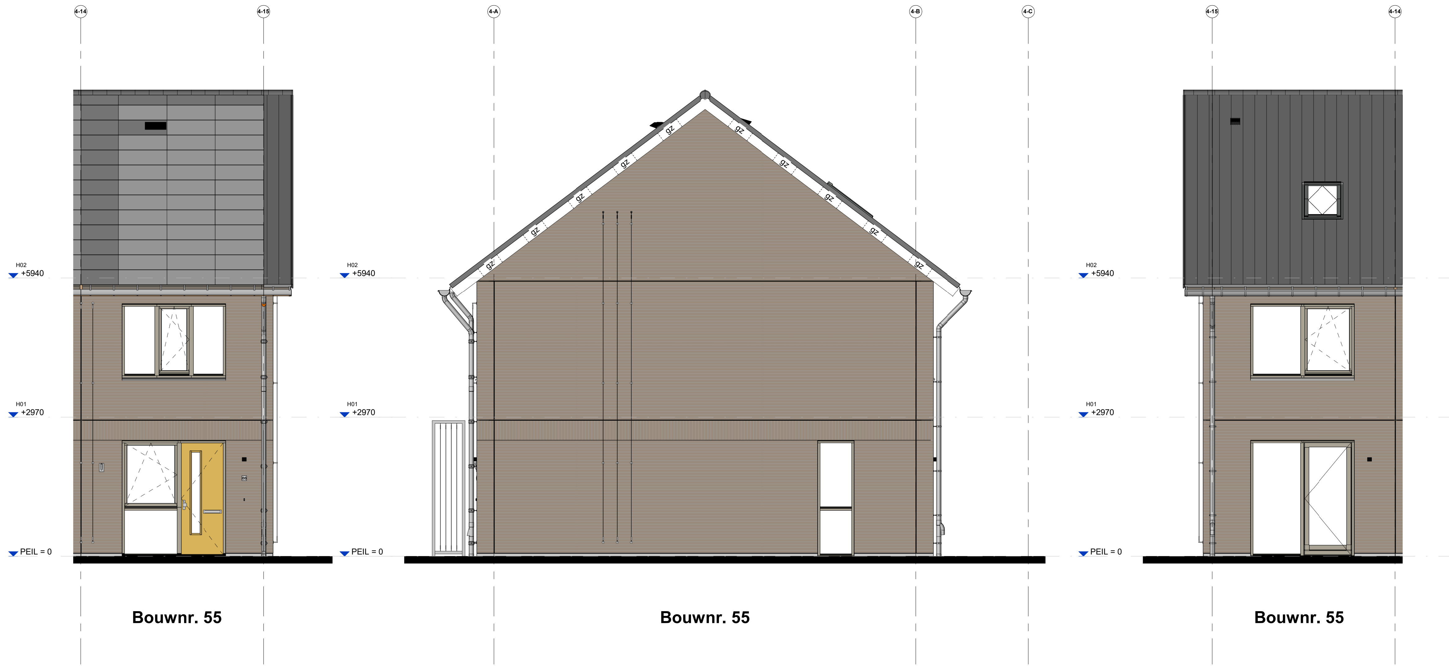
Voorgevel
