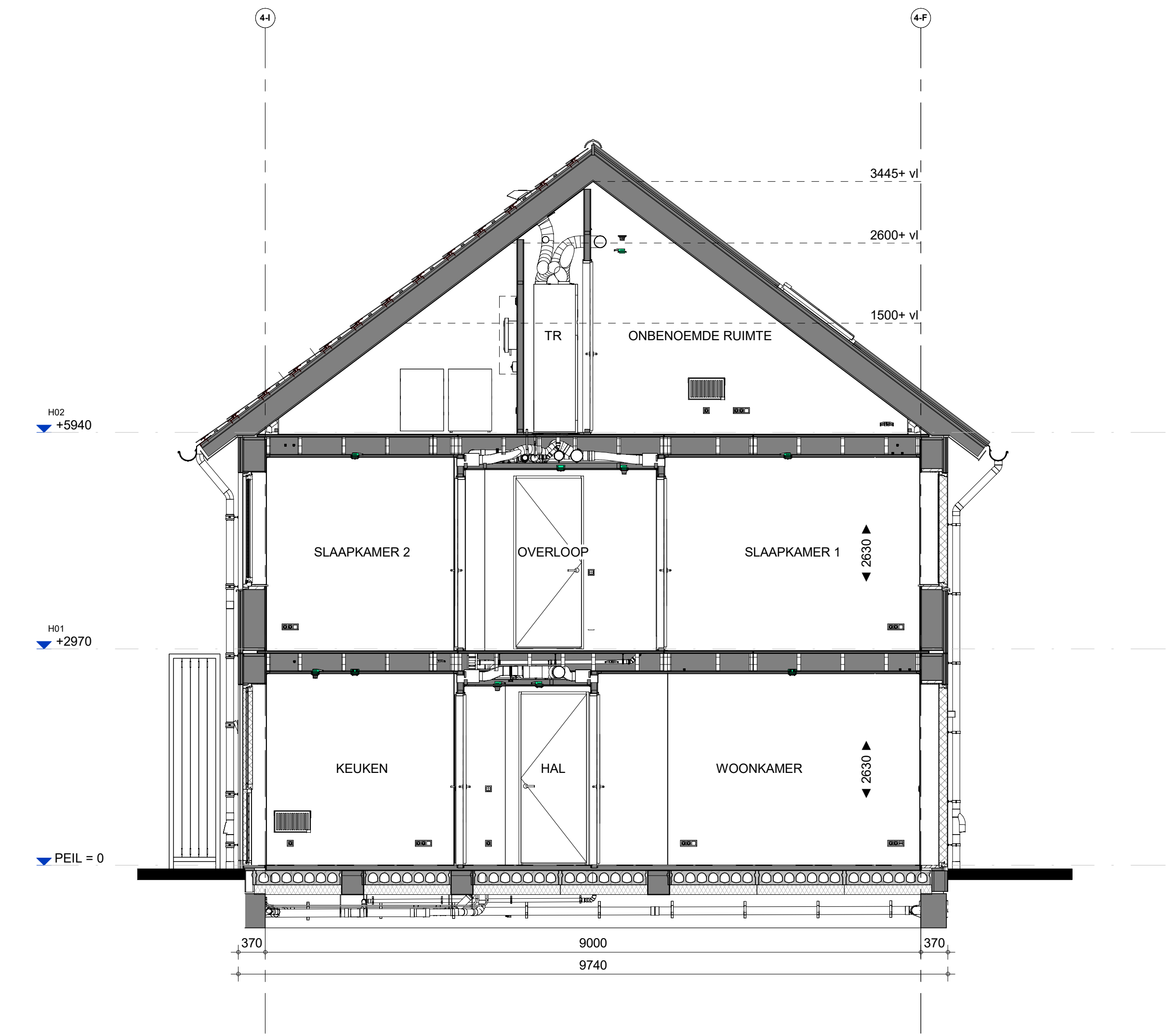
Doorsnede
