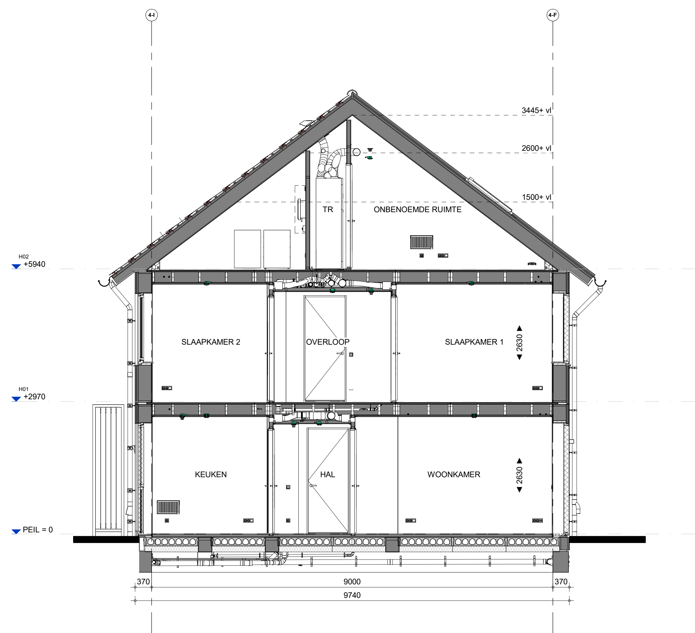
Doorsnede
