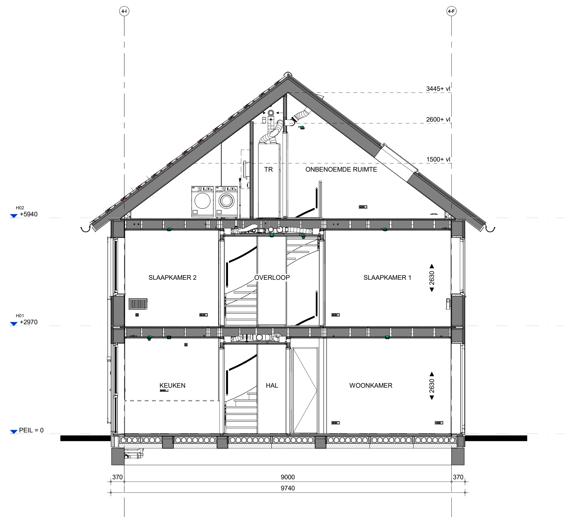
Doorsnede
