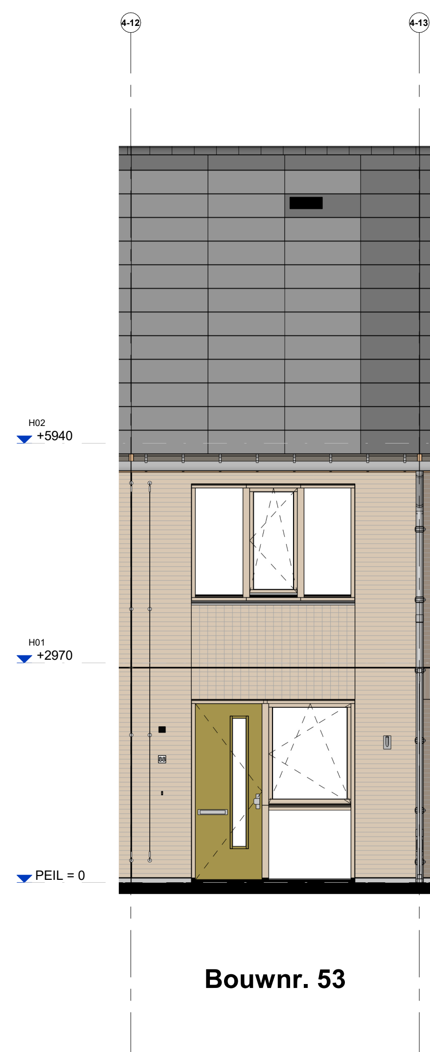
Voorgevel
