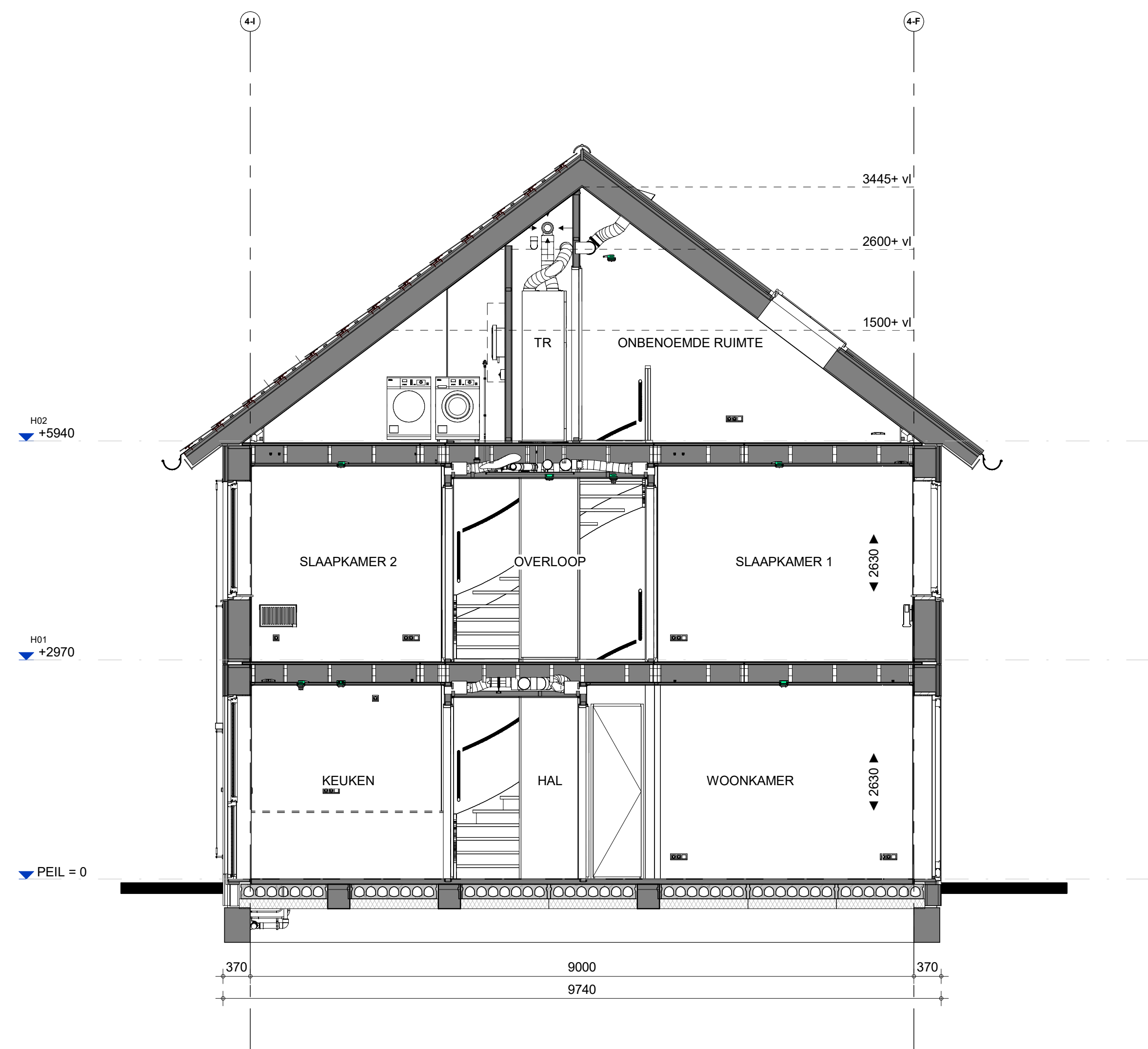
Doorsnede
