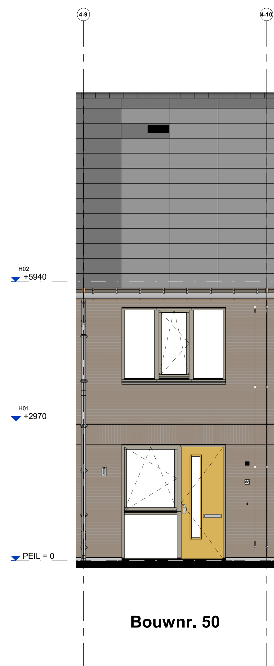
Voorgevel
