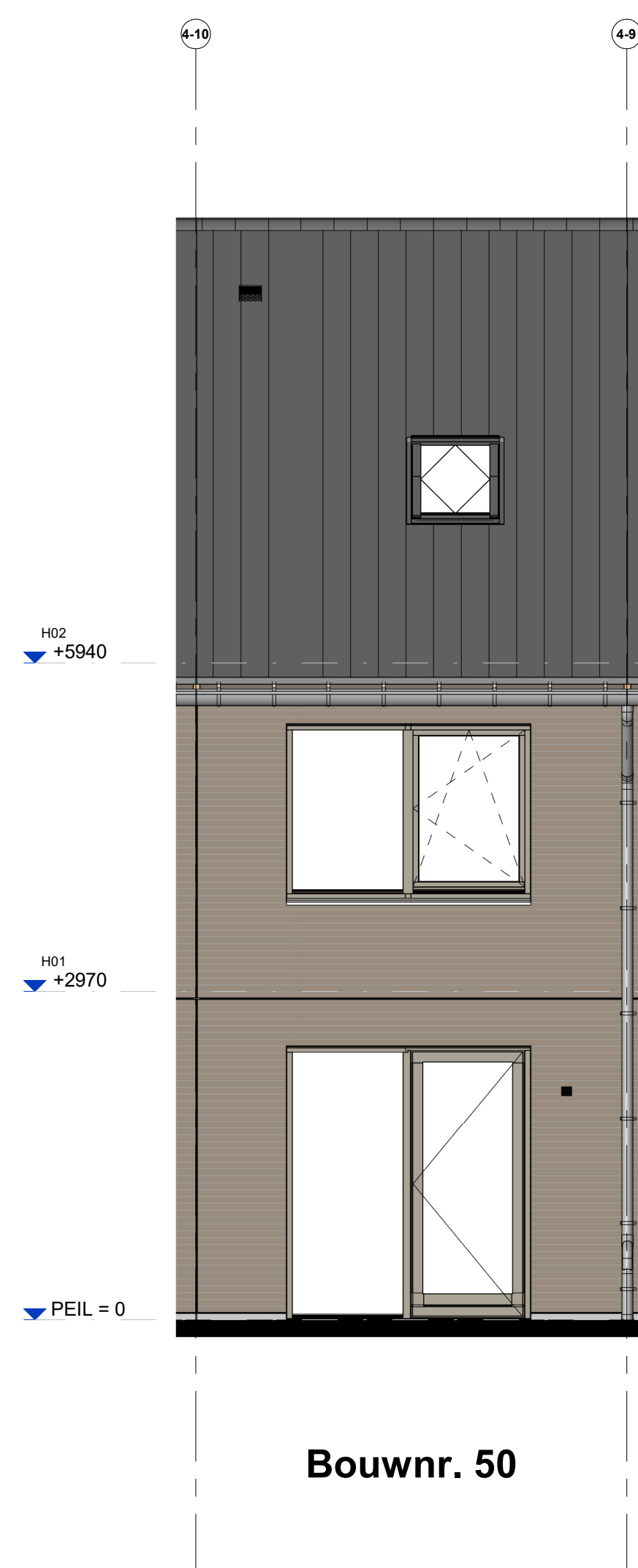
Achtergevel
