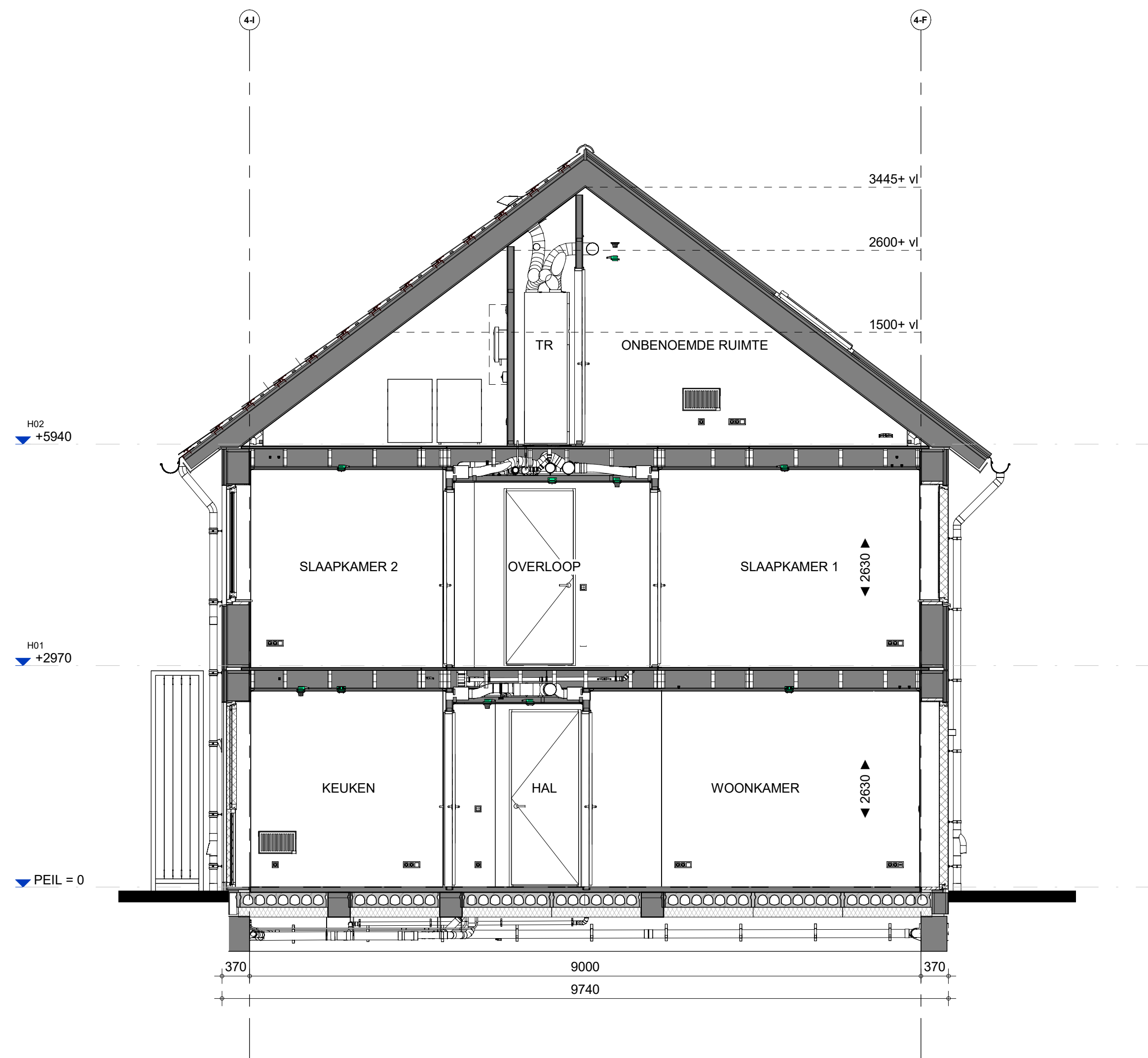
Doorsnede
