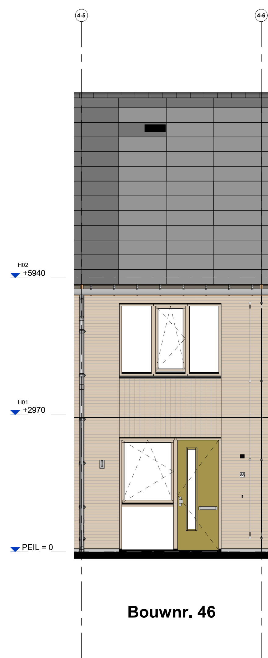
Voorgevel
