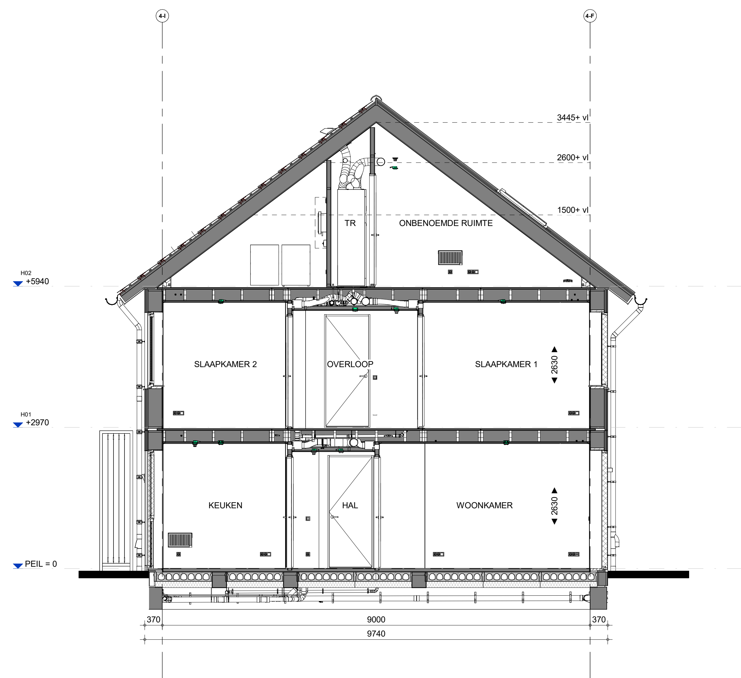
Doorsnede
