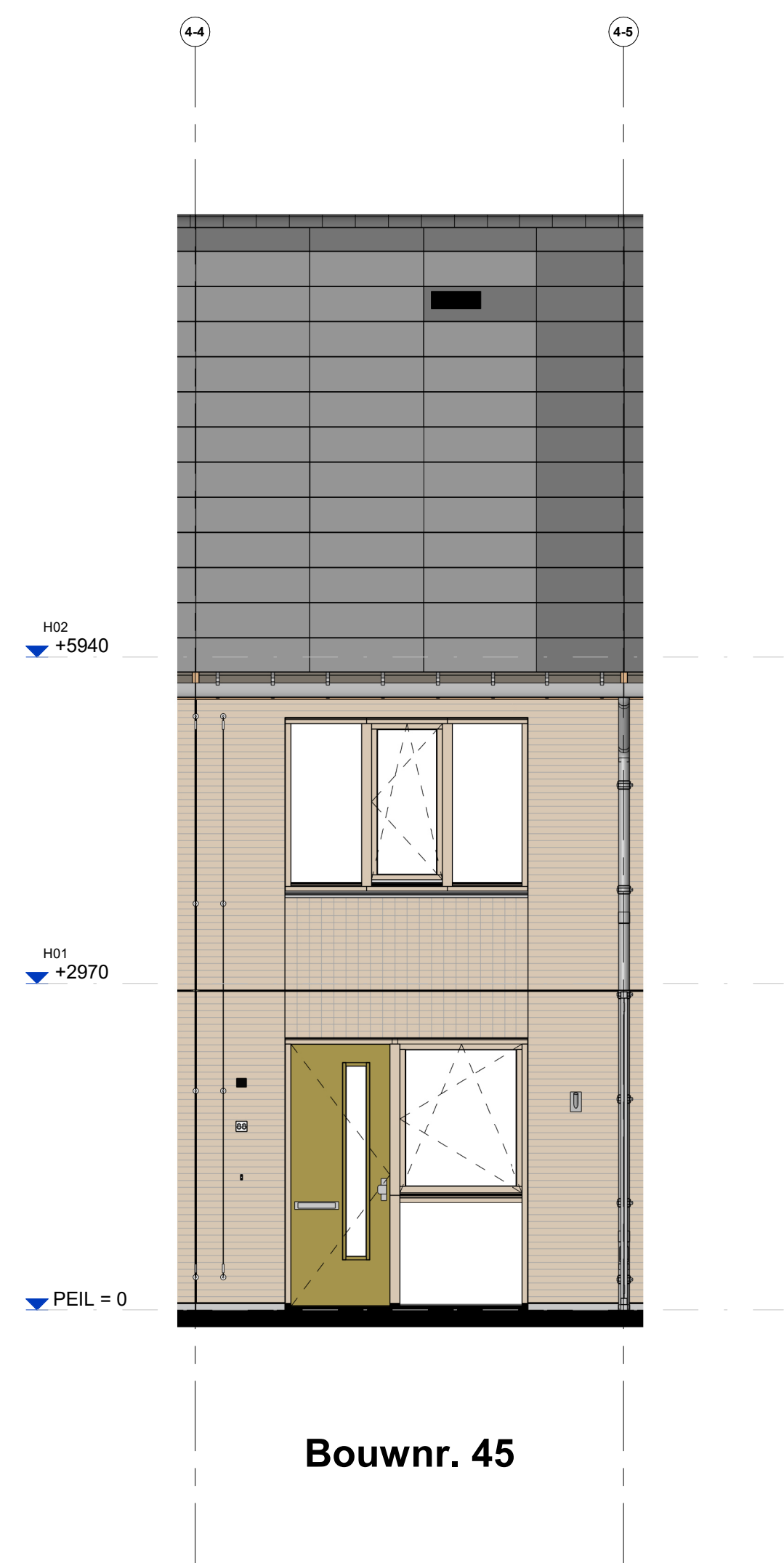
Voorgevel
