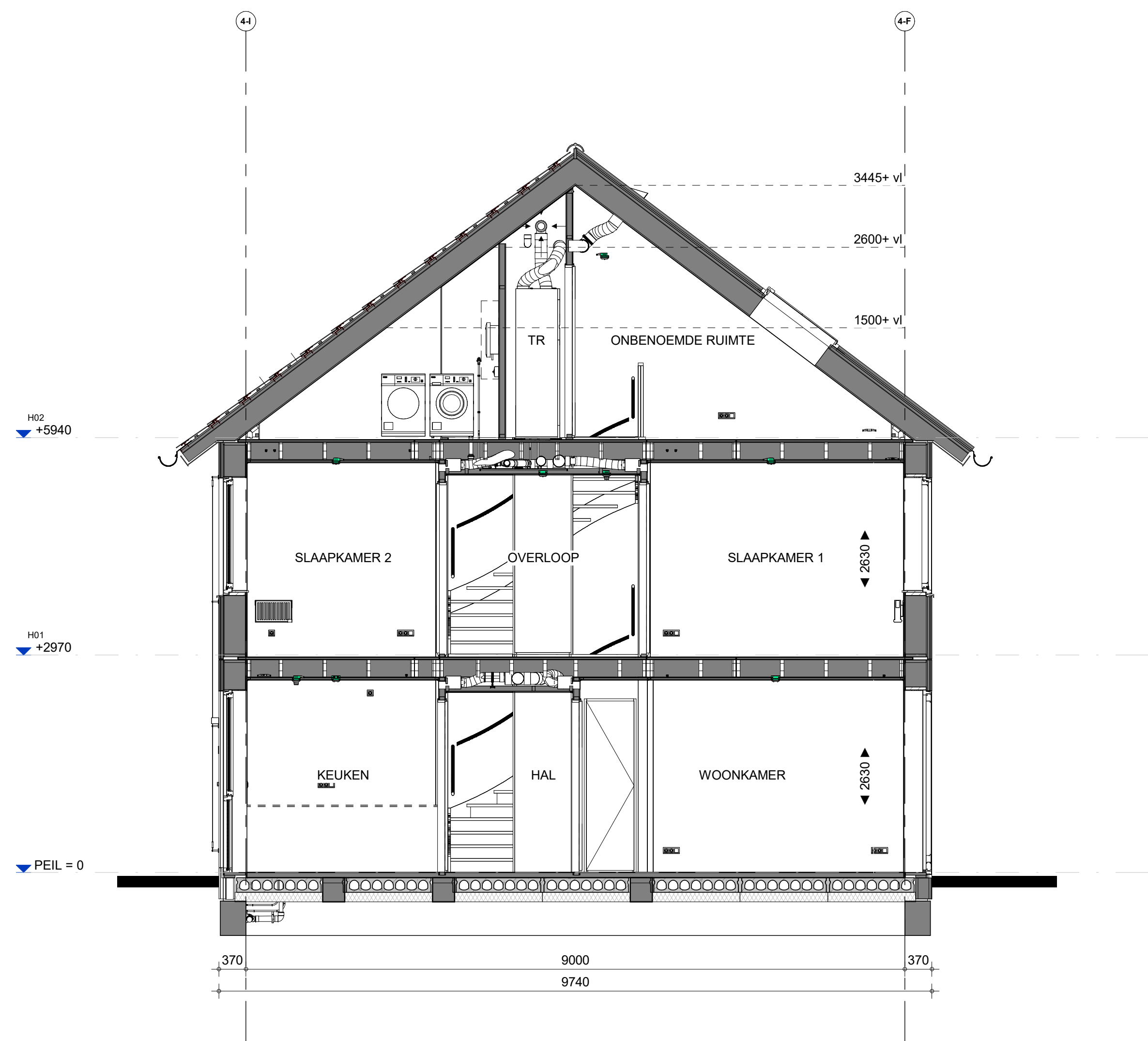
Doorsnede
