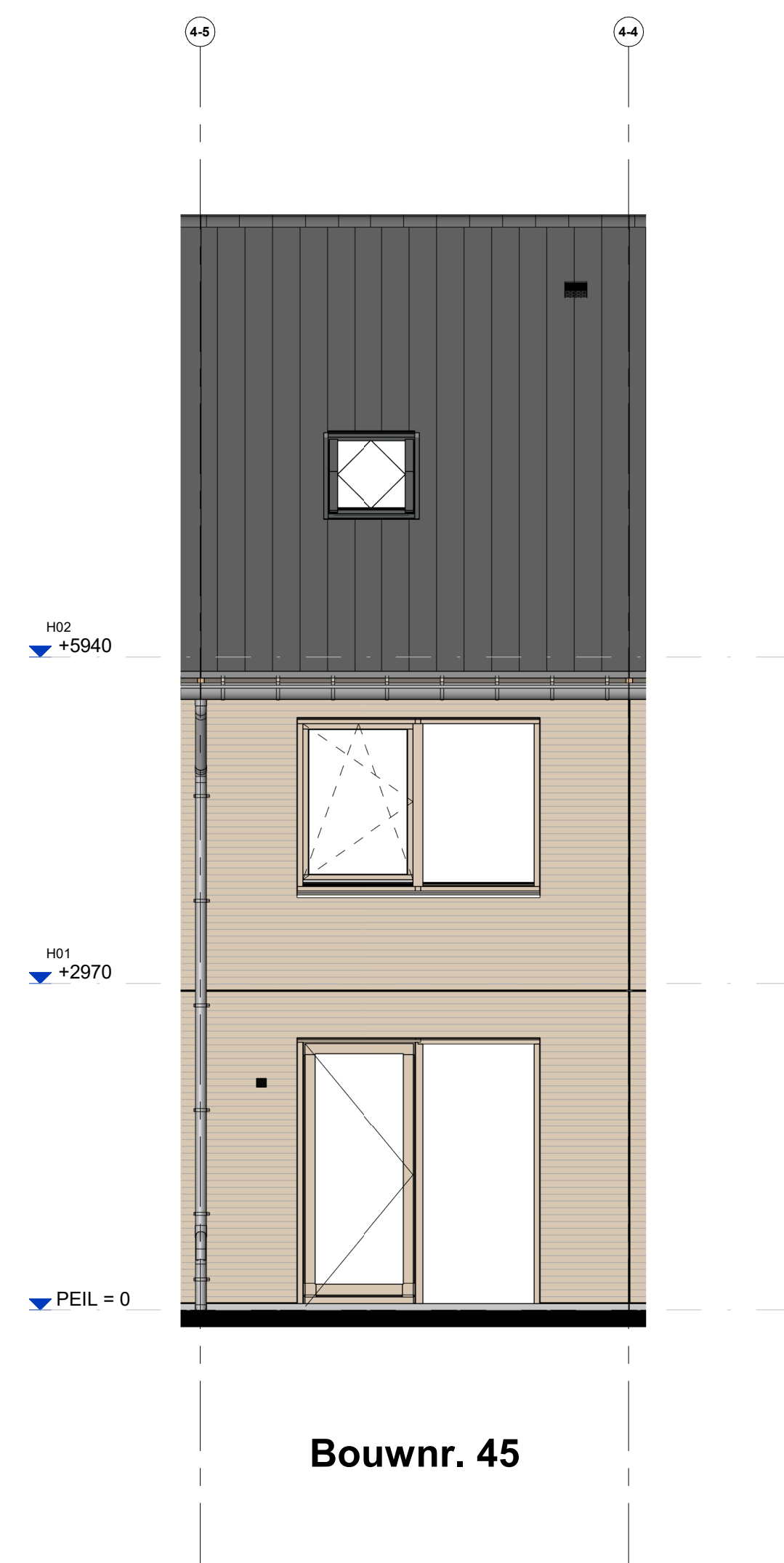
Achtergevel
