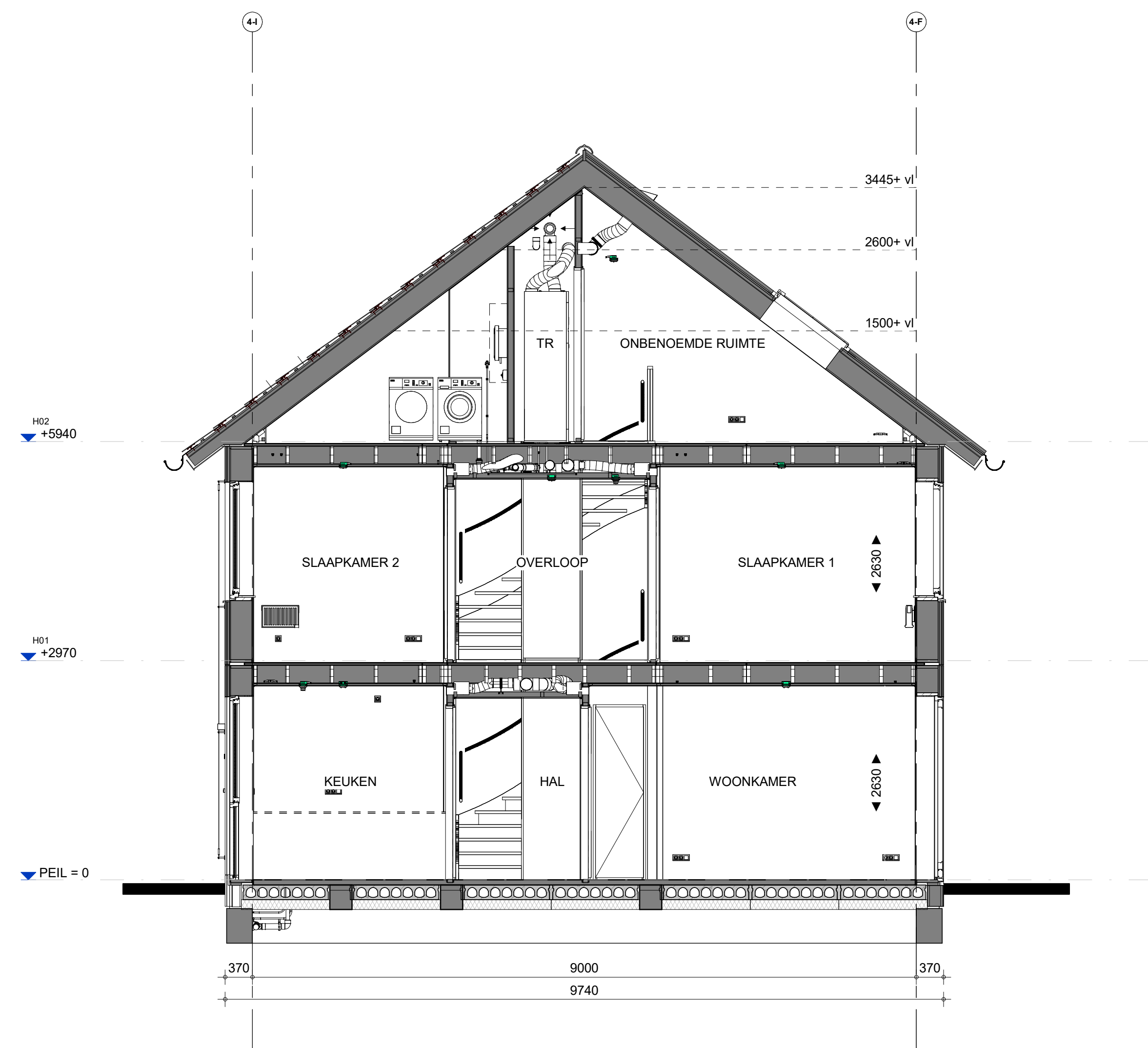
Doorsnede
