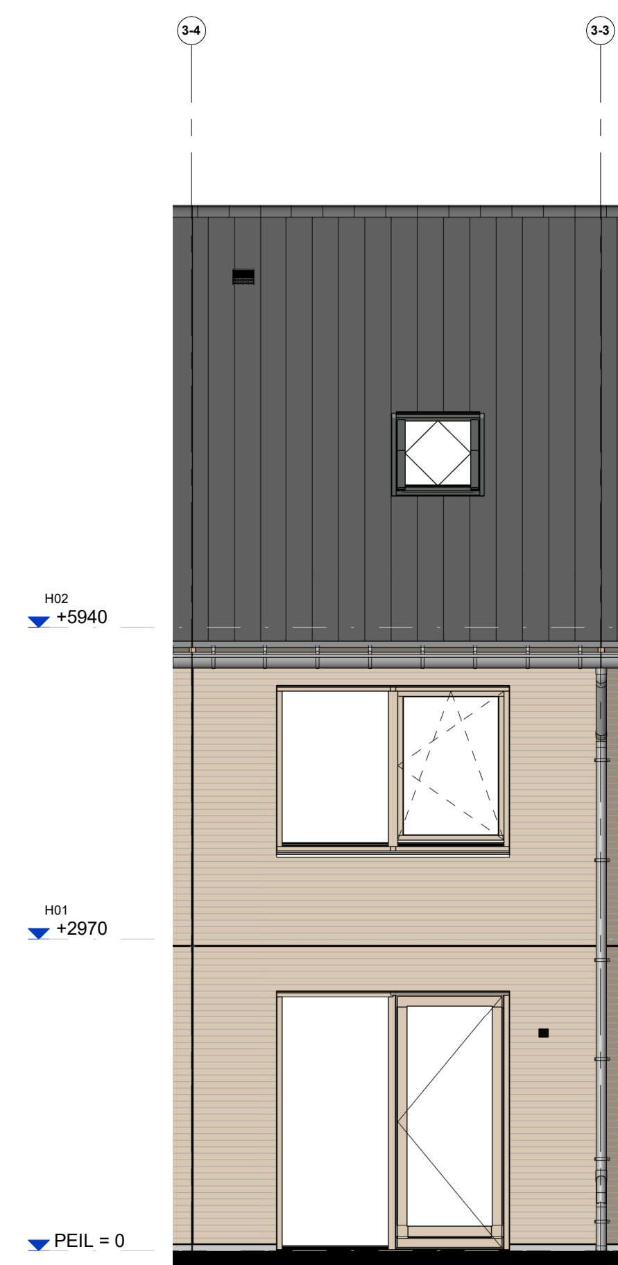
Bouwnr. 39
