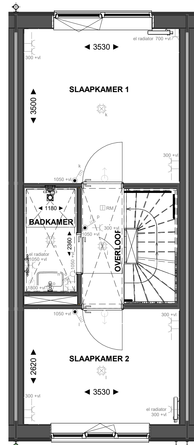
Bouwnr. 39
