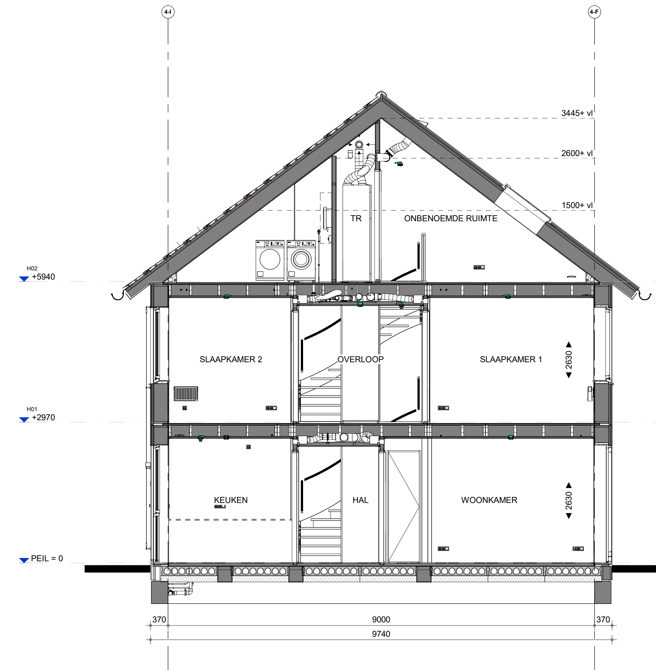
Doorsnede
