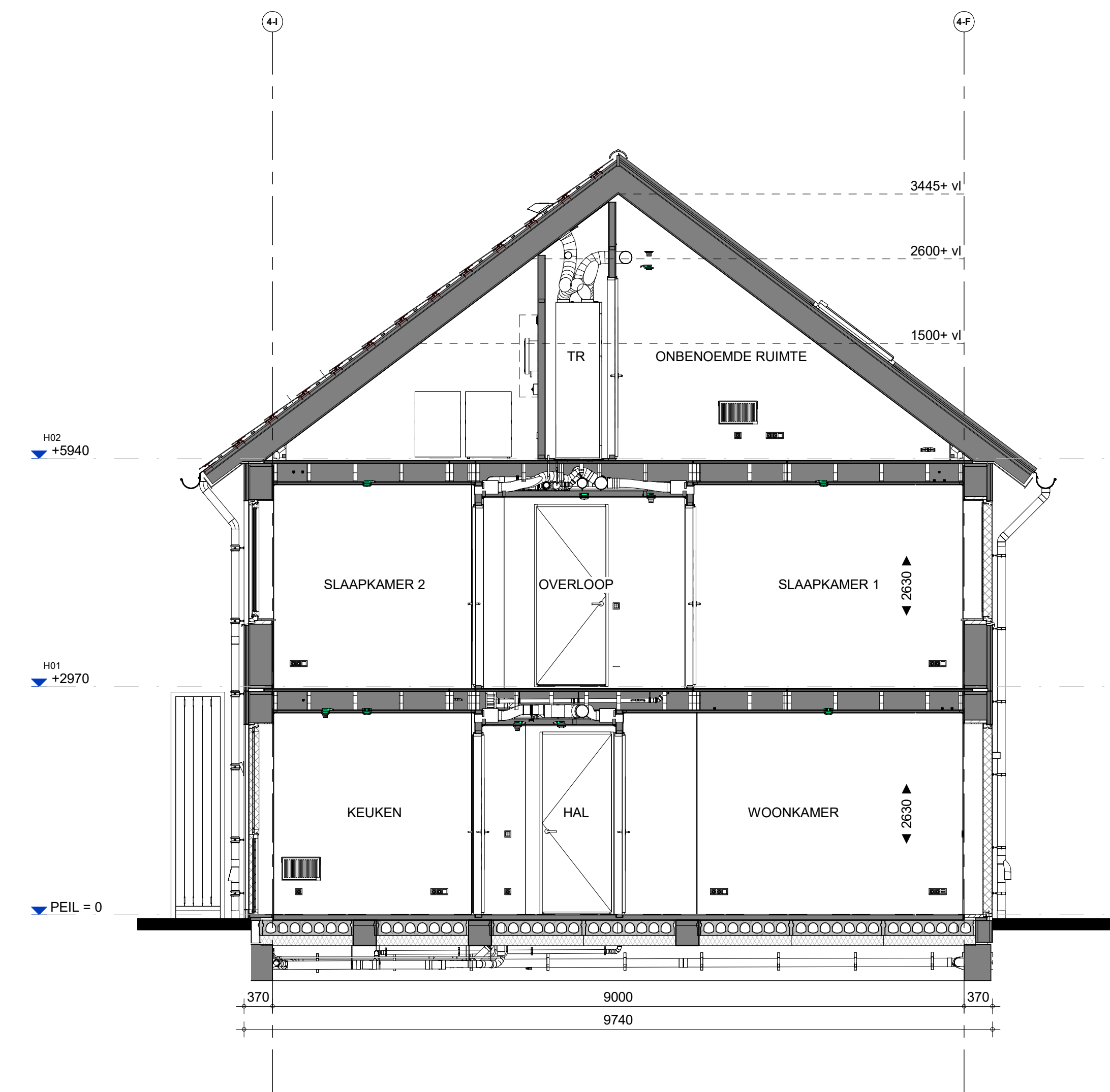
Doorsnede
