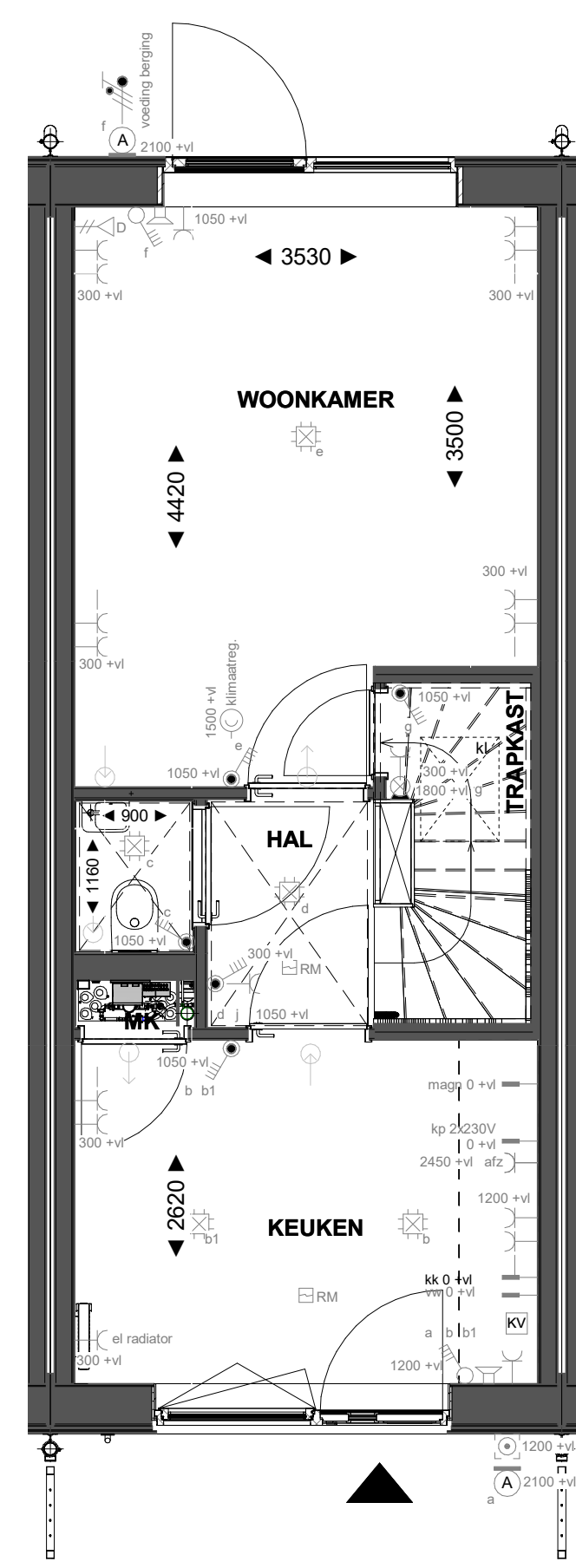
Begane grond
