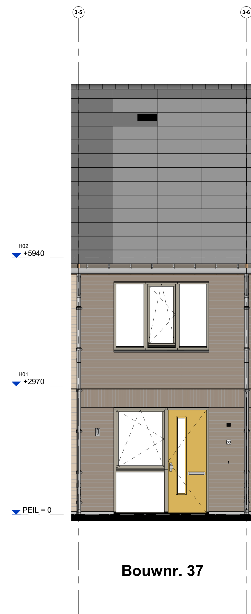
Voorgevel
