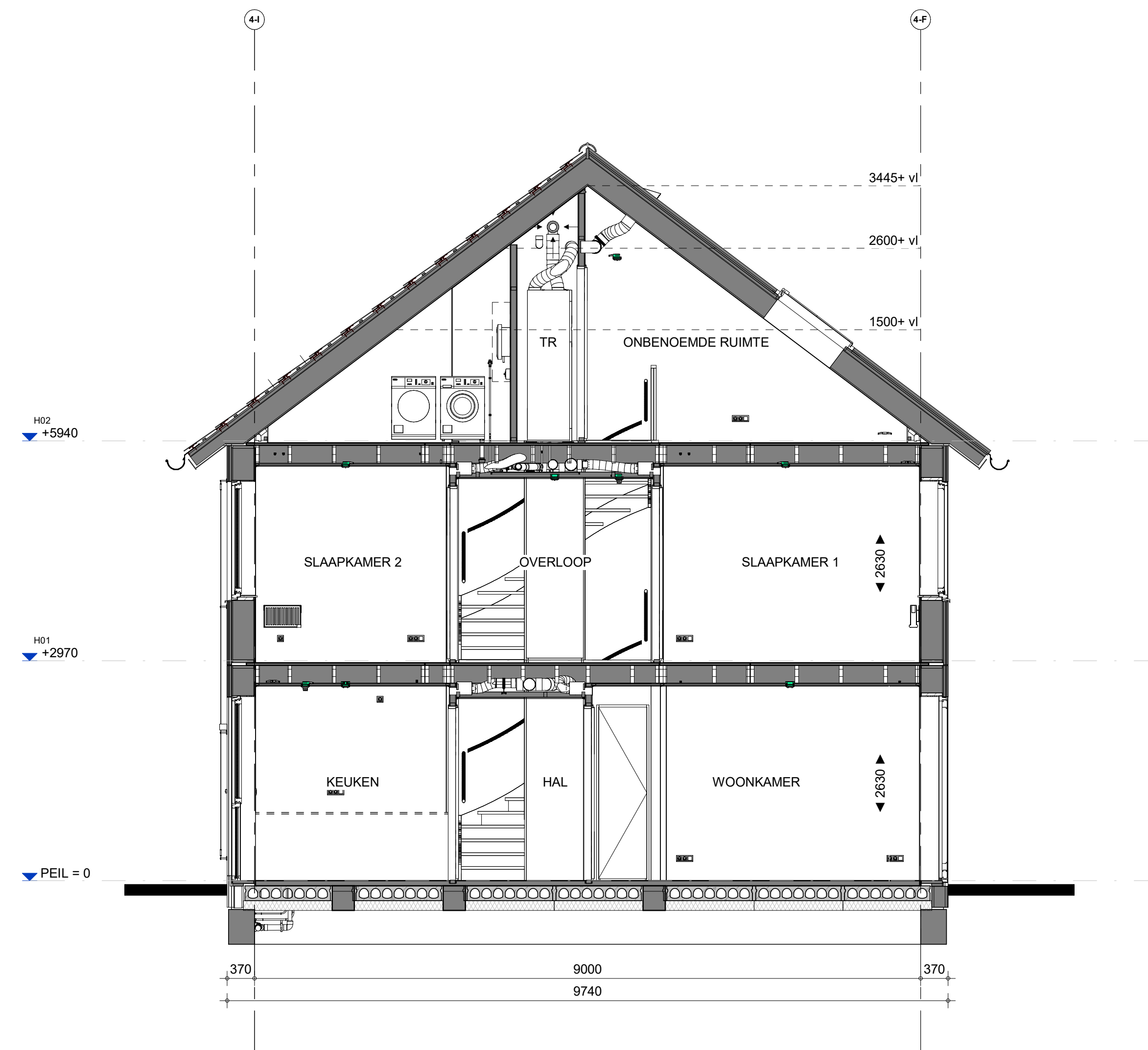
Doorsnede
